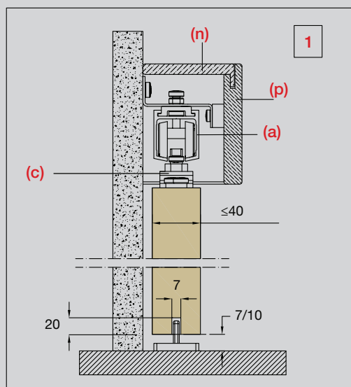
A) Instalación en la pared sin rodapié, para paneles de grosor (SP) \leq 40 mm. Installation sur la cloison sans plinthe, pour panneaux portes avec épaisseur (SP) \leq 40 mm
