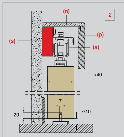
B) Instalación en la pared con rodapié, para paneles de grosor (SP) > 40 mm. Installation sur la cloison avec plinthe, pour panneaux portes avec épaisseur (SP) > 40 mm
